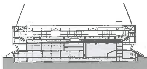
Querschnitt Fussballstadion.
