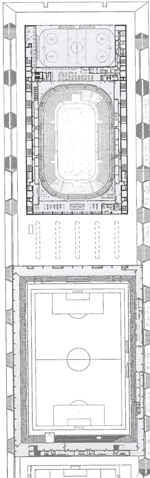
Grundriss mit Eishalle, Eishockeystadion, «place publique» und Fussballstadion.
