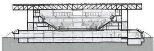
Querschnitt Eishockeystadion. 0 25 50m
